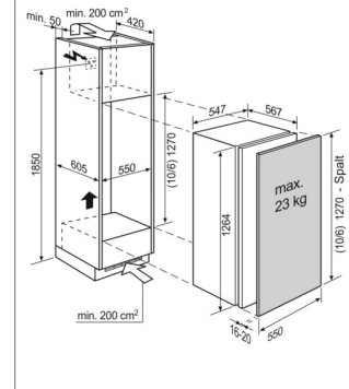
IK247S / IK245S / IK243S Möbelfront auf Gerätetür verschraubt
