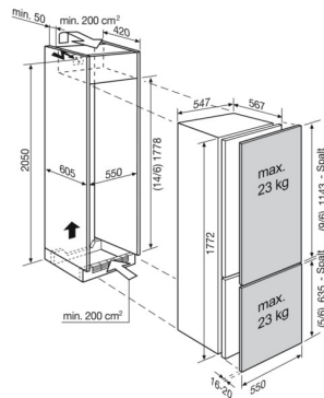
IK309BN / IK307BN / IK305BN Möbelfronten auf Gerätetüren verschraubt
