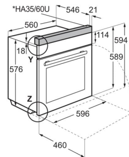
Einbaubackofen/Einbauberherd + Höhenadapter EB6.../EH6... + HA35/60U
